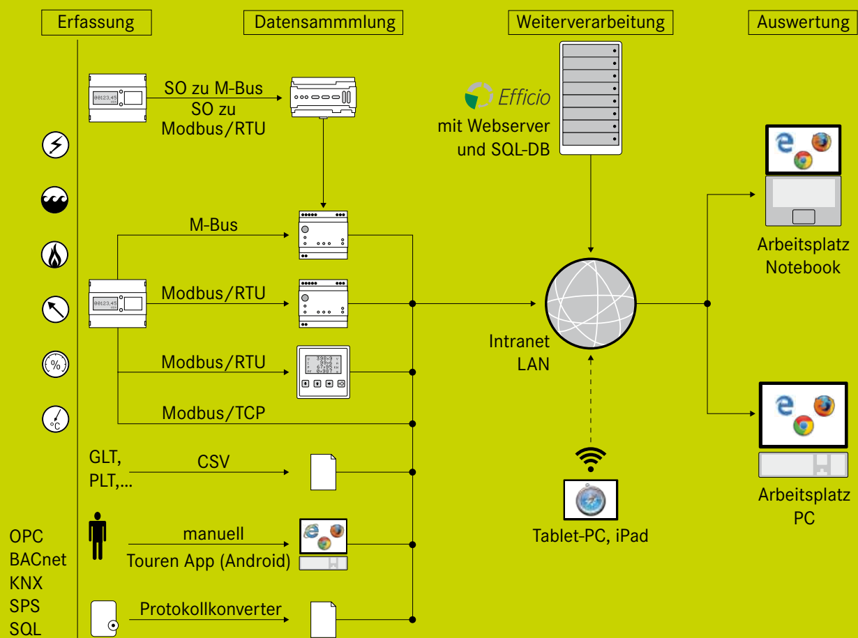
Systemaufbau Efficio
